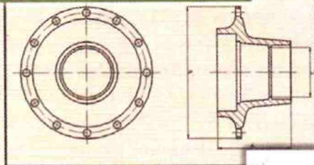
Креслення
