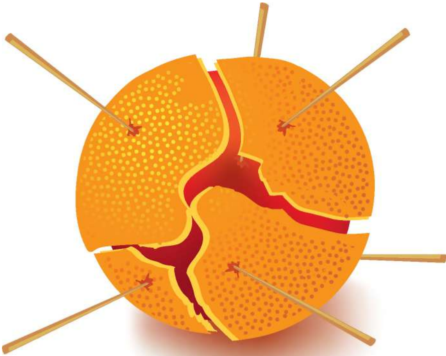
Модель земної кори
