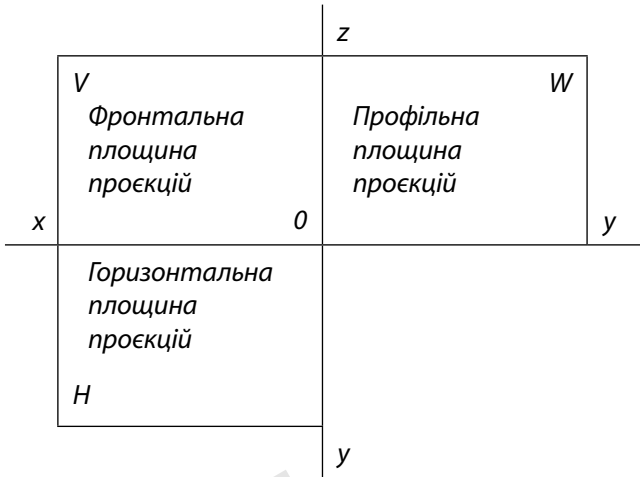
Мал. 3.8. Розташування площин проєкцій
