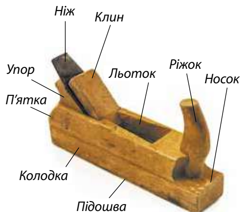
Мал. 6.2. Будова рубанка
