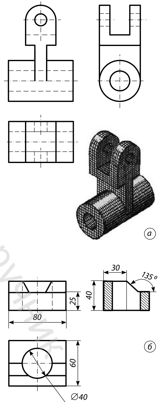
Мал. 3.9. Розташування виглядів на кресленику
