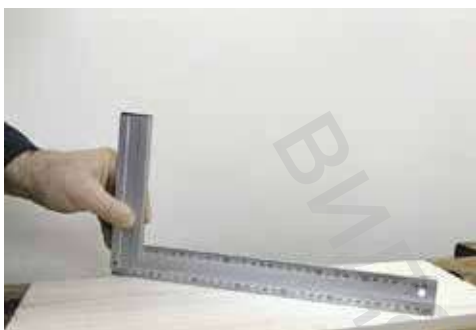
Мал. 6.9. Перевірка стругання площини лінійкою та кутником
