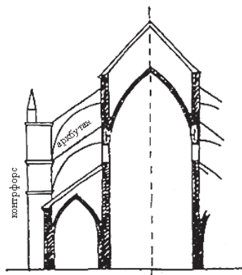
Структура готичного собору у поперечному розрізі
