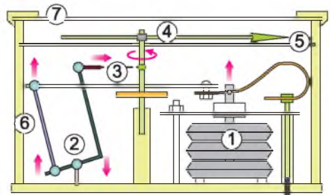
Схема барометра-анероїда
