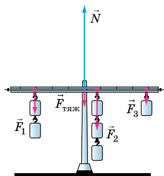
Рис. 2.3. Важіль залишається нерухомим, якщо справджується правило моментів, а сили, що діють на важіль, скомпенсовані
