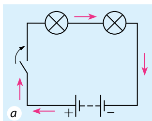
Рис. 34.4. Схеми деяких електричних кіл: а — схема послідовного з'єднання двох ламп (див. рис. 34.3, а ); б — схема паралельного з'єднання двох ламп (див. рис. 34.3, б ). Стрілками позначено напрямки струму в разі замкнення ключа
