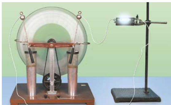
Рис. 33.2. Якщо різнойменно заряджені кондуктори електрофорної машини з'єднати з електричною лампою, у лампі виникне електричний струм. Лампа світитиметься, доки обертаються диски машини, — у цьому випадку механічна енергія перетворюється на електричну
