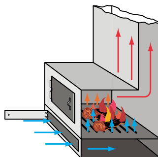
Рис. 14.6. Створення тяги: збагачене киснем холодне повітря потрапляє до печі завдяки конвекції
