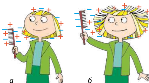
Рис. 29.2. Перед розчісуванням кількість позитивних зарядів на волосся й гребінці дорівнює кількості негативних (а). Під час розчісування частина електронів з волосся перейде на гребінець, унаслідок чого гребінець зарядиться негативно, а волосся — позитивно (б)
