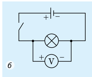
Рис. 36.2. Вимірювання вольтметром напруги на лампі: а — загальний вигляд; б — схема електричного кола
