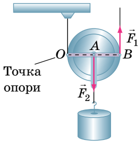
Рис. 3.4. Рухомий блок можна розглядати як важіль, у якого відношення плечей становить 1:2
