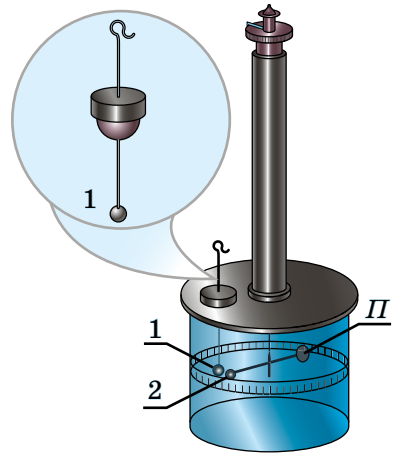
Рис. 30.2. Принцип дії крутильних терезів Кулона. На тонкому дроті закріплено коромисло, на кінцях якого розміщені кулька 2 і протипава П. Крізь отвір у кришці скляного циліндра опускають заряджену кульку 1
