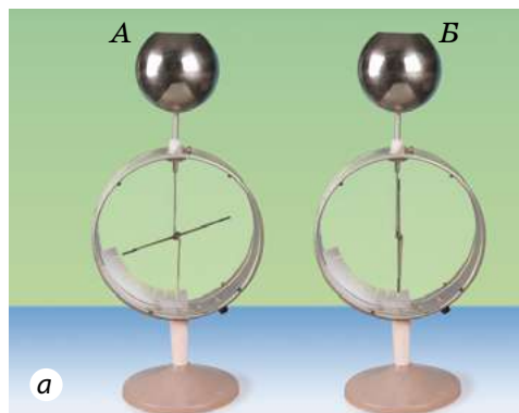
Рис. 31.1. Якщо заряджений електрометр з'єднати з незарядженим за допомогою провідника, частина заряду перейде на незаряджений електрометр
