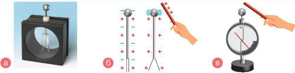
Мал. 19.7. Електроскоп (а), принцип дії електроскопа (б), електрометр (в)
