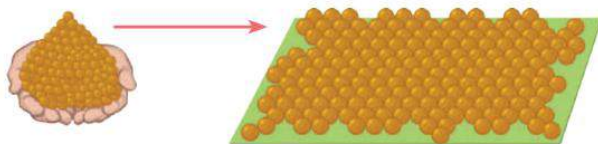
Мал. 1.9. Моделювання молекулярного шару
