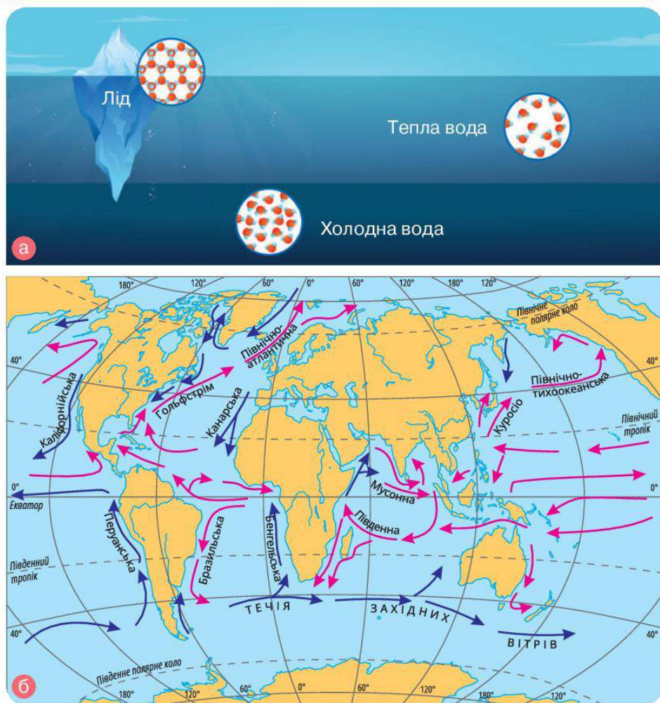
Мал. 4.3. а — розширення води при замерзанні;
