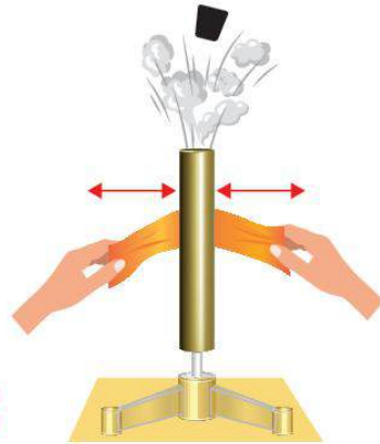
Мал. 5.2. Що є причиною зміни внутрішньої енергії в кожному випадку?
