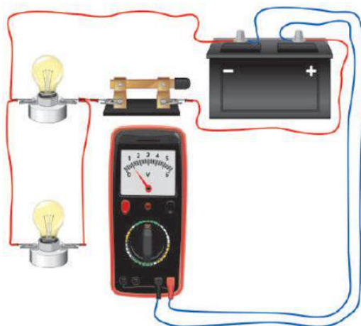
Мал. 28.1. Вимірювання напруги в колі з паралельним з'єднанням провідників: а — на джерелі; б — на першій лампі; в — на другій лампі
