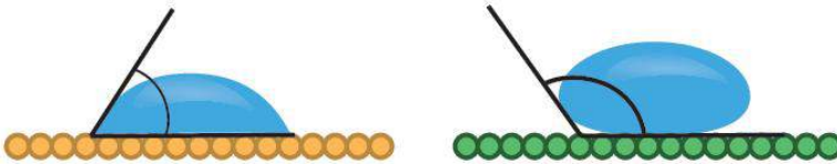
Мал. 9.4. а — рідина змочує поверхню; б — рідина не змочує поверхню
