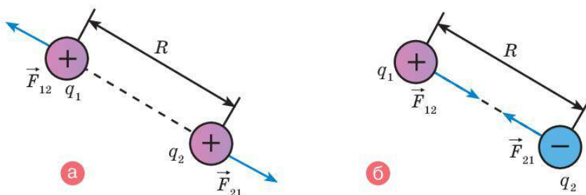
Мал. 20.3. Напрями сил взаємодії точкових зарядів:
