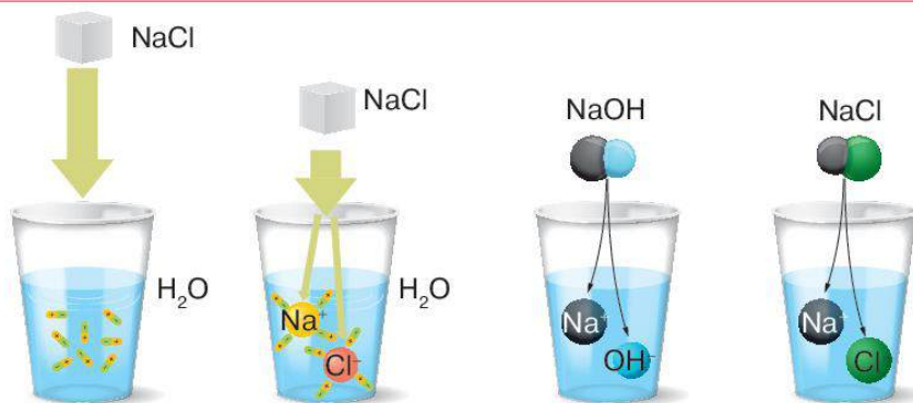
Мал. 31.2. У розчині утворюються вільні носії електричного струму
