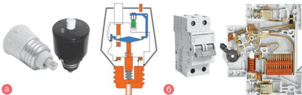
Мал. 32.4. Запобіжники: а — одноразові; б — автоматичні (багаторазові)
