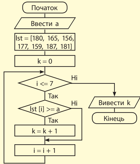
Рис. 13.15. Блок-схема алгоритму визначення кількості учнів, які вступили на факультет (до прикладу 1)
