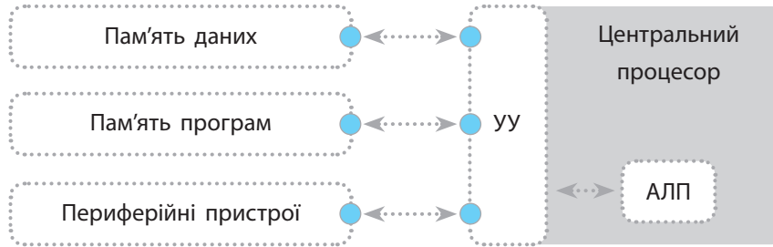
Рис. 3.11. Схема ЕОМ за Гарвардською архітектурою
