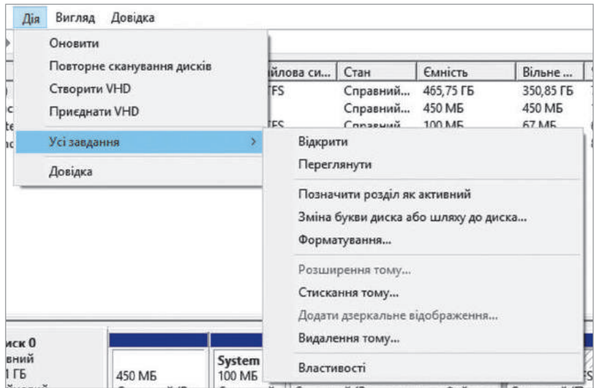
Рис. 3.45. Вигляд вікна з командами списку Усі завдання
