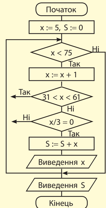
Рис. 13.18. Блок-схема алгоритму визначення чисел, кратних 3, та їх суми (до прикладу 2)
