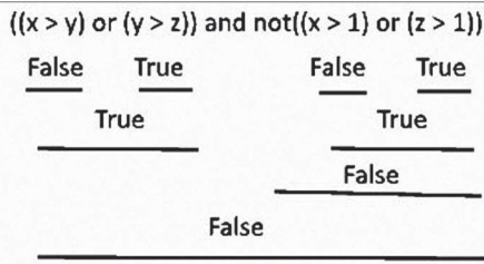
Рис. 11.1. Аналіз значення логічного виразу
