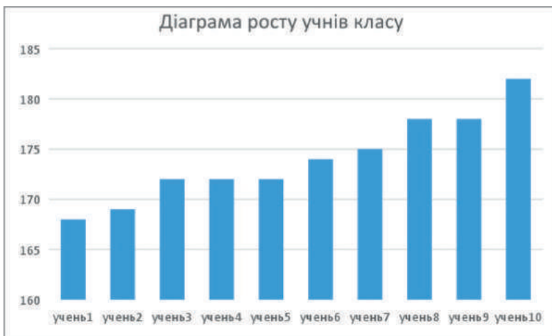
Рис. 7.17. Гістограма аналізу зросту учнів
