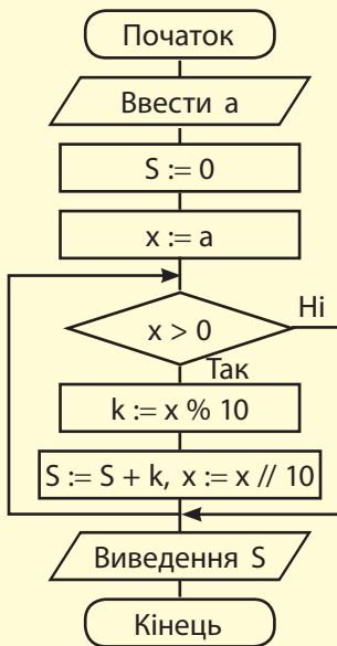
Рис. 13.8. Блок-схема алгоритму обчислення суми цифр
