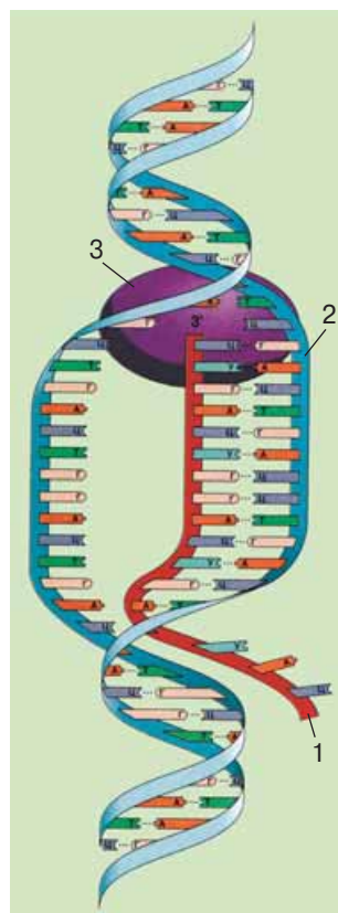
Мал. 12.2. Процес самоподвоєння молекули ДНК: за участі ферменту розшиваються водневі зв'язки (1) і на кожному материнському ланцюзі за принципом комплементарності добудовується дочірній (2)
