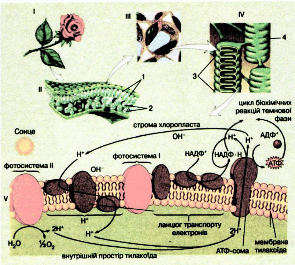
Мал. 28.1. Структури, які забезпечують фотосинтез: I – фотосинтезуюча рослина; II – зріз через листову пластинку; зверніть увагу на стовпчасти (1) та губчасті (2) клітини, в яких розташовані хлоропласти; III – внутрішня будова рослинної клітини; IV. Деталі будови хлоропласта: окремі тилакоїди (4) та грани (3); V – процес перенесення електронів під час фотосинтезу
