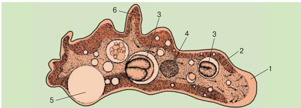
Мал. 19.1. Схематична будова клітини амеби: 1 – шар ектоплазми; 2 – шар ектоплазми; 3 – травні вакуолі; 4 – ядро; 5 – скоротлива вакуоля; 6 – псевдоподія (стрілки на малюнку вказують напрямок руху цитоплазми)
