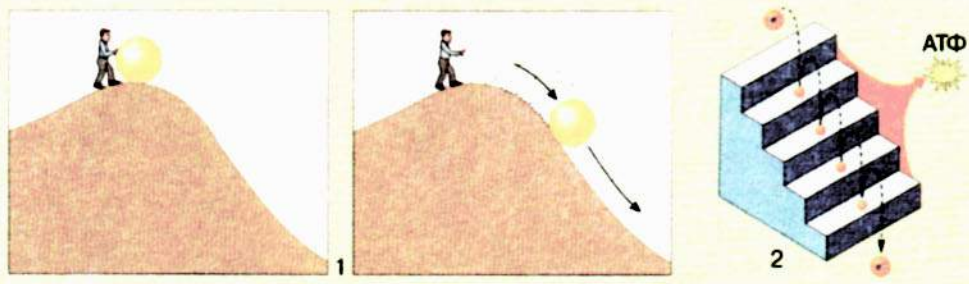
▶ Мал. 28.2. 1. Схема, що ілюструє перетворення потенційної енергії в кінетичну. Коли людина піднімає кулю на гору, вона надає їй потенційної енергії. Коли куля котиться з гори, вона віддає цю енергію. Ця енергія розсіюється. 2. Те саме відбувається з електроном: коли він переходить на вищий енергетичний рівень, то отримує потенційну енергію. Коли ж за допомогою ланцюга перенесення електронів він повертається на нижчий рівень, то віддає цю енергію. Частина енергії розсіюється у вигляді тепла, однак вона переважно запасається у вигляді макроергічних зв'язків молекул АТФ
