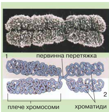
Мал. 18.2. 1. Фотографія хромосоми, зроблена за допомогою електронного мікроскопа. 2. Схема будови хромосоми
