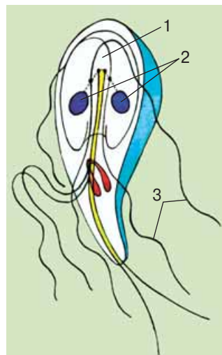
Мал. 19.3. Клітина лямблїї: 1 – опорний стрижень; 2 – ядра; 3 – джгутики
