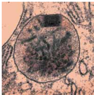
Мал. 20.7. Одномембрanna органела – пероксисома
