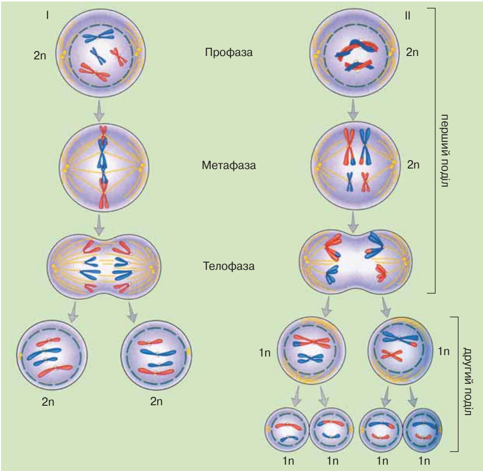
Мал. 25.5. Розбіжності між мітозом (I) і мейозом (II)
