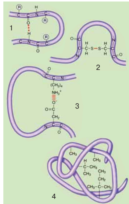
Мал. 9.2. Зв'язки, які підтримують конформації білкової молекули: 1 – водневі; 2 – дисульфідні; 3 – йонні взаємодії; 4 – гідрофобні взаємодії
