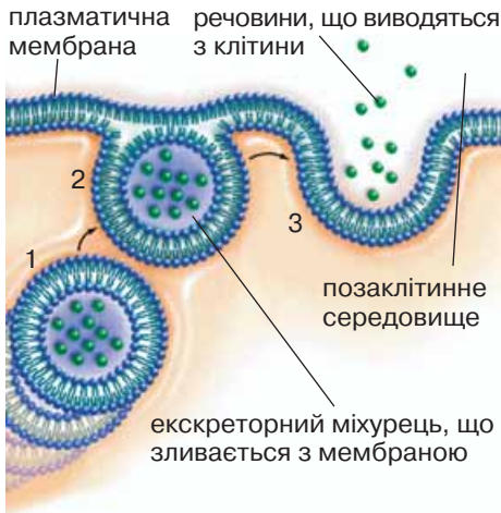
Мал. 15.7. Послідовні стадії екзоцитозу (1–3)
