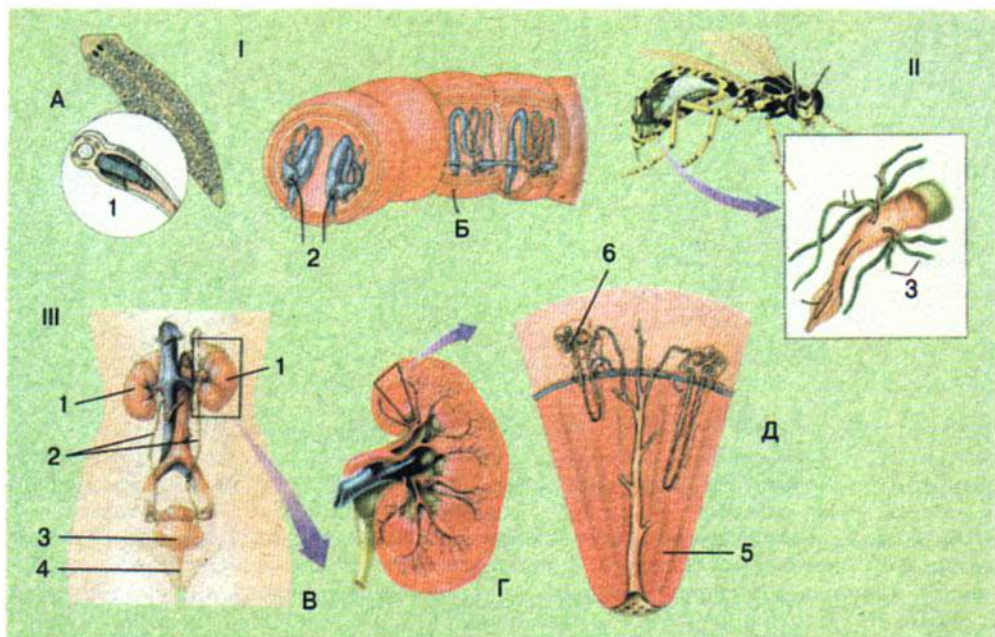
Мал. 43.9. I. Видільна система плоских (А) та кільчастих (Б) червів (1 – протонефридії плоских червів; 2 – метанефридії кільчастих). II. Видільна система членистоногих представлена мальпігієвими судинами (3). III. Видільна система людини: В – план будови; 1 – нирки; 2 – сечоводи; 3 – сечовий міхур; 4 – сечівник. Г – нирка в розрізі; Д – ниркова пірамідка (5) з нефронами (6)
