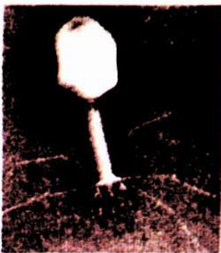
Мал. 30.6. Електронно-мікроскопічна фотографія віріона бактеріофага T4
