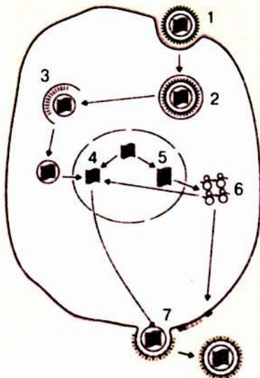
Мал. 32.2. Життєвий цикл вірусу грипу: 1 – приєднання вірусу до чутливої клітини; 2 – утворення ендосоми (пухирця) з вірусом; 3 – злиття мембран і потрапляння РНК вірусу в цитоплазму; 4 – проникнення РНК вірусу до ядра клітини; 5 – транскрипція і реплікація вірусної РНК; 6 – синтез вірусних структурних білків та збирання віріонів; 7 – «вихід» віріонів з клітини
