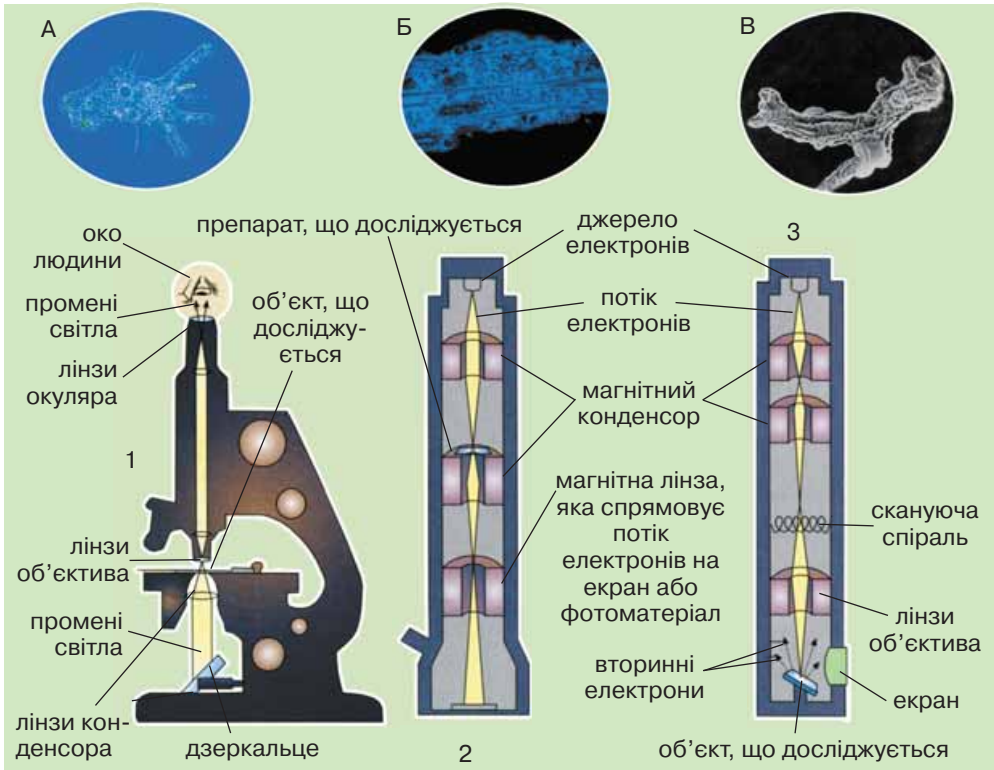
Мал. 14.3. Фотографії амеби, зроблені за допомогою: А – світлового мікроскопа; Б – електронного мікроскопа; В – сканувального мікроскопа. Принцип роботи світлового (1), електронного (2) та сканувального (3) мікроскопів
