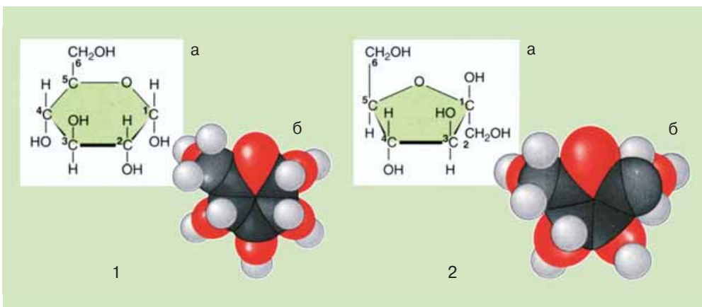
Мал. 8.1. Моносахариди глюкоза (1) і фруктоза (2): а – хімічна формула; б – просторова модель
