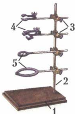
Мал. 19. Лабораторний штатив
