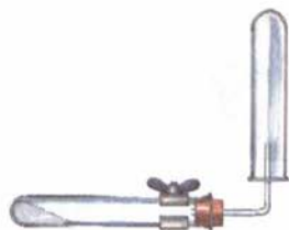
Мал. 48. Наповнення посудини газоподібними речовинами, легшими за повітря
