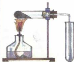
Мал. 55. Добування кисню з калій перманганату та збирання його витісненням повітря
