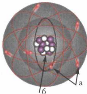
Мал. 25. Модель атома Карбону: а — електрони, б — ядро атома
