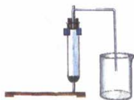
Мал. 49. Добування кисню з гідроген пероксиду
