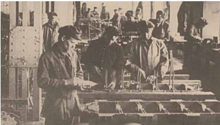
Монтаж двигуна М-6 у складальному цеху. Завод авіадвигунів ДЕКА. Олександрівськ. 1916 р.
