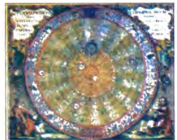
Рис. 3. Система Коперника
