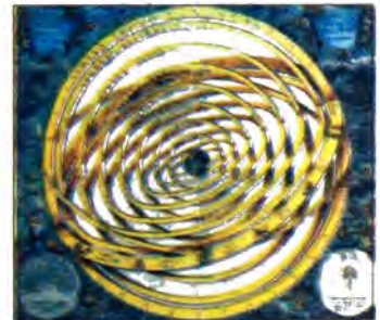
Рис. 2. Система Птолемея
